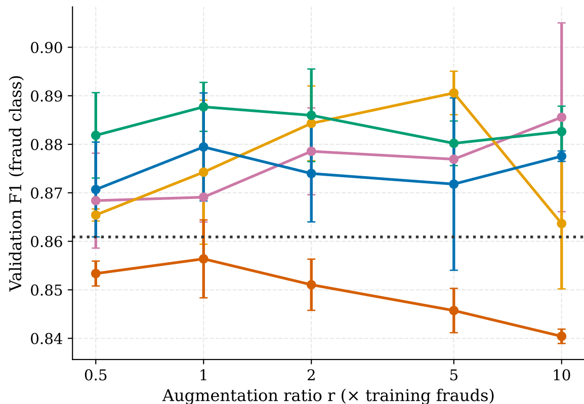
MLP
